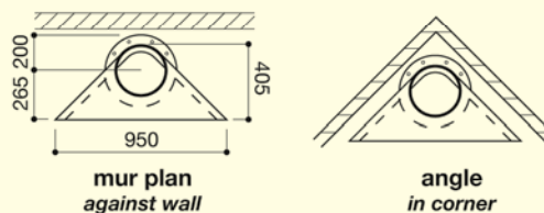
vues de dessus - plan views
